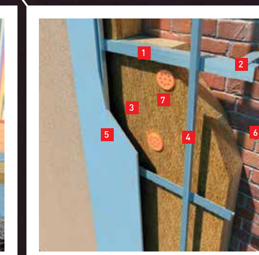
Навесной вентилируемый фасад
