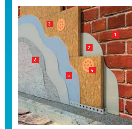
Штукатурный фасад
