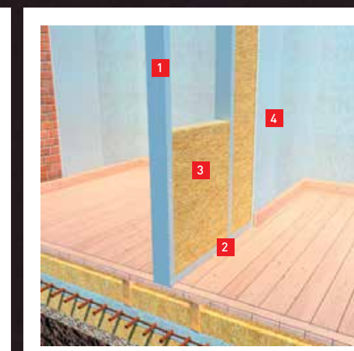
Перегородки
