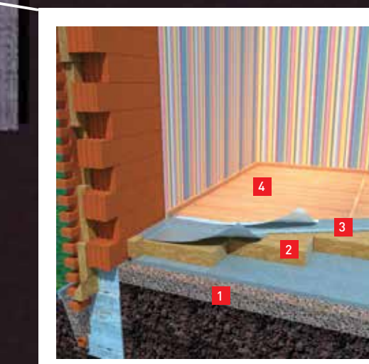
Полы по грунту
